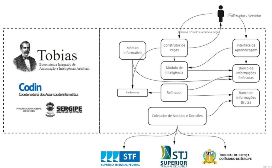
Diagrama TOBIAS; Fonte: Codin
